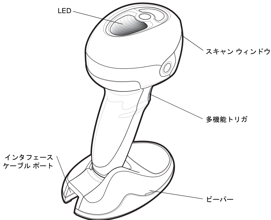
図 2-1 パーツ
