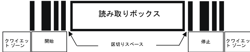
図 I-2 CapCode の構造
