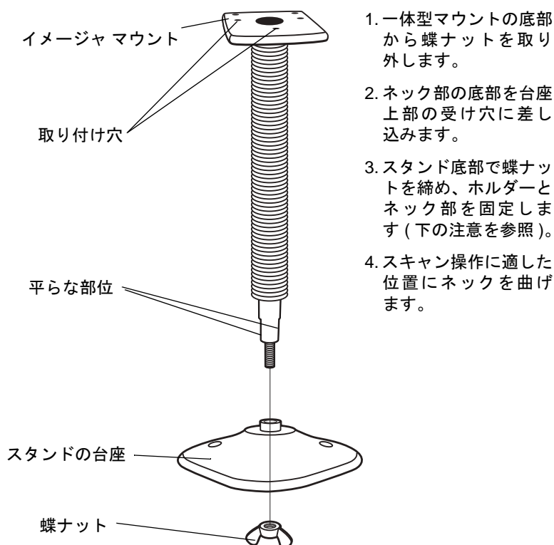
図2-2 ゲースネック スタンドの組み立て
