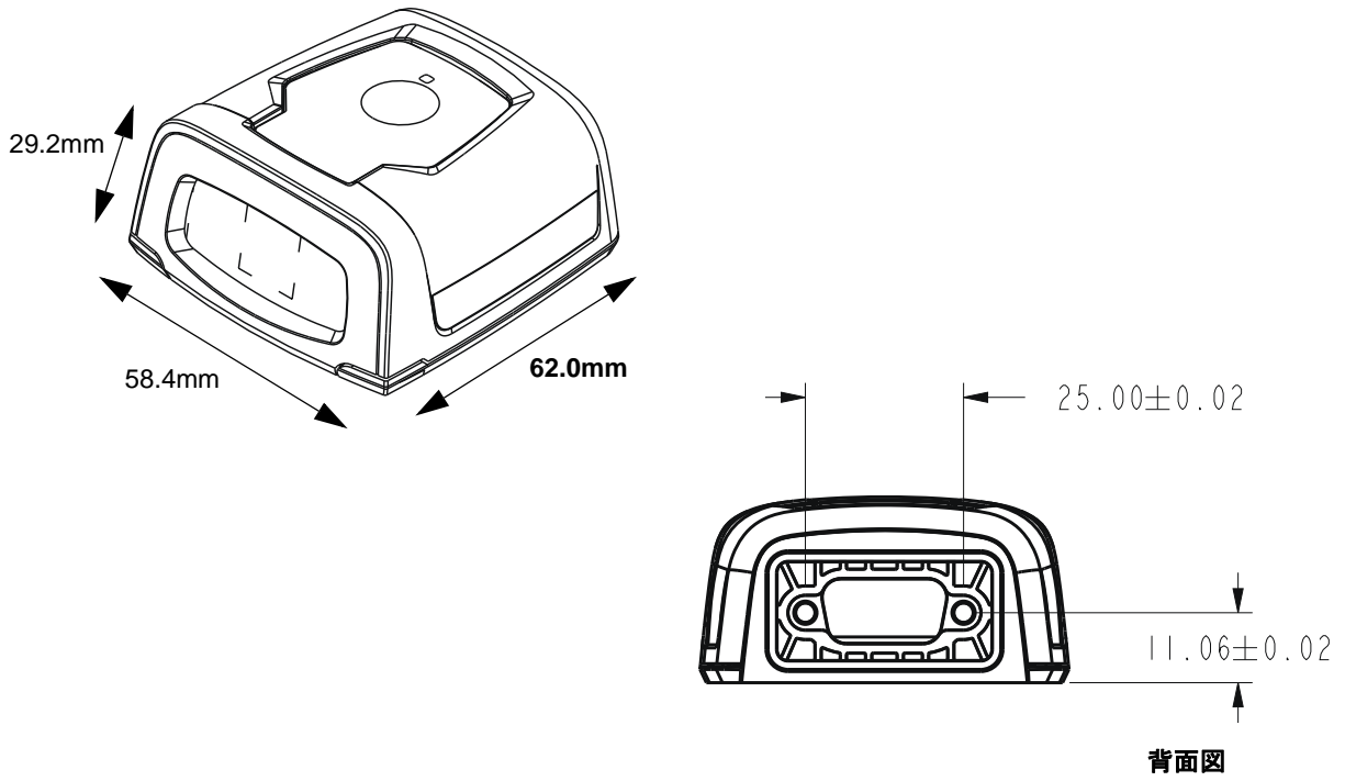
図 4-2 DS457 の寸法図
