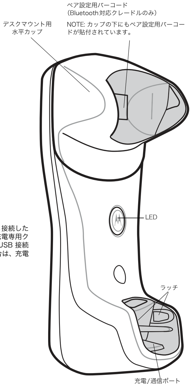
図1-2 シングルスロットクレードル - 接続部とペア設定用バーコード
