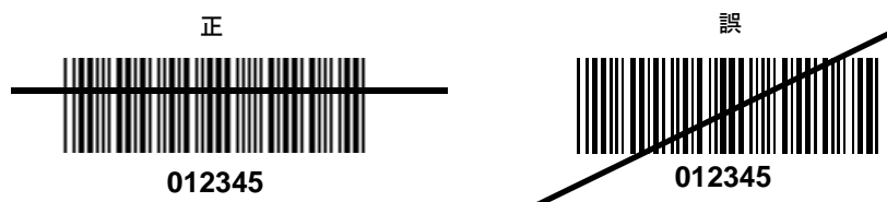
図3-5 シンボルの向きとレーザスキヤナの照準パターン
