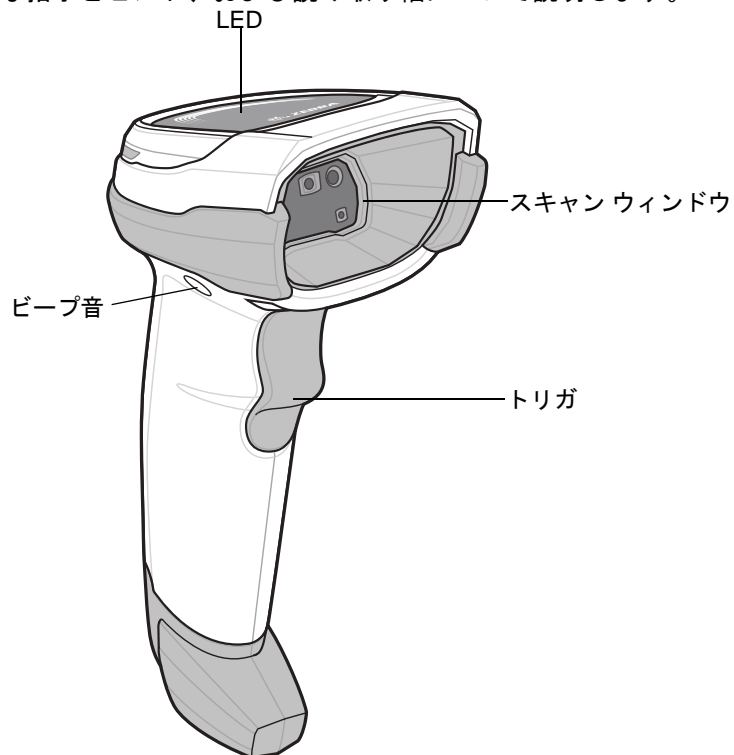
図 2-1 DS8108 の構成部品
