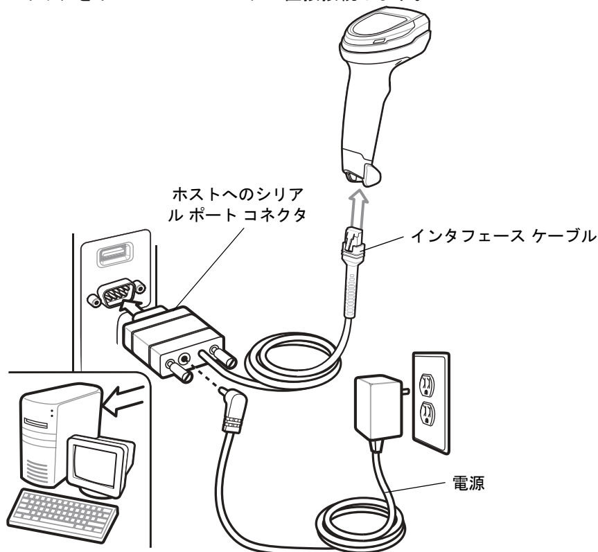
図 6-1 RS-232 接続
