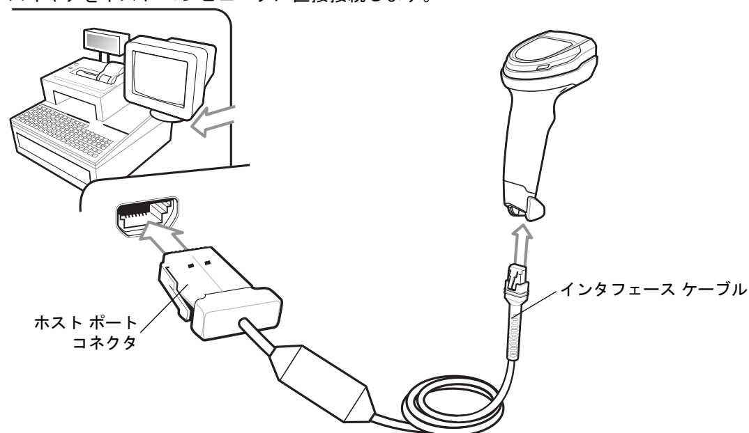
図 7-1 IBM 接続
