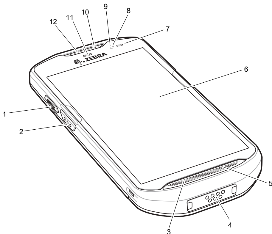
図1 TC56 正面図
