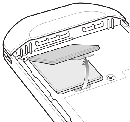
図23 アクセスドアの取り外し
