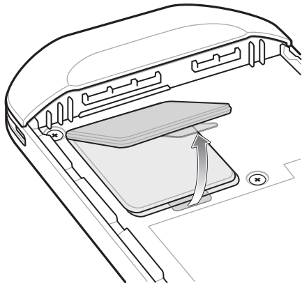
図20 アクセスドアの取り外し
