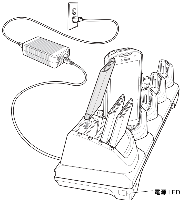
図 134 予備バッテリーの充電
