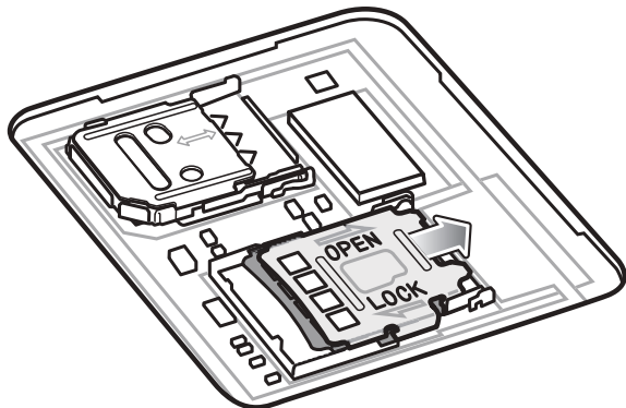
図6 SIM カードホルダーを持ち上げる
