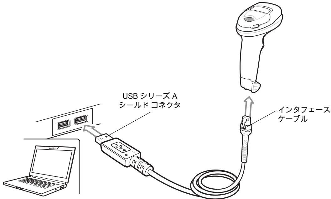
図 13 USB 接続
